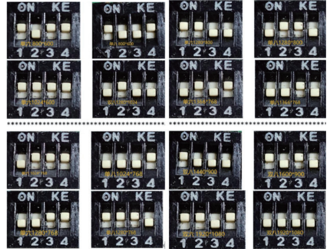
LVDS分辨率拨码：SW1
