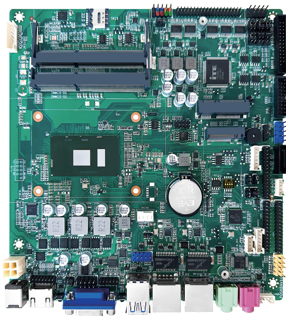
正面图
