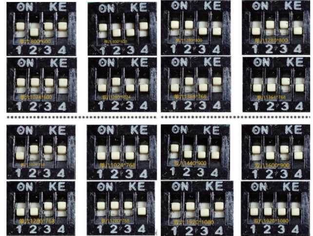
拨码开关LVDS分辨率示意图
