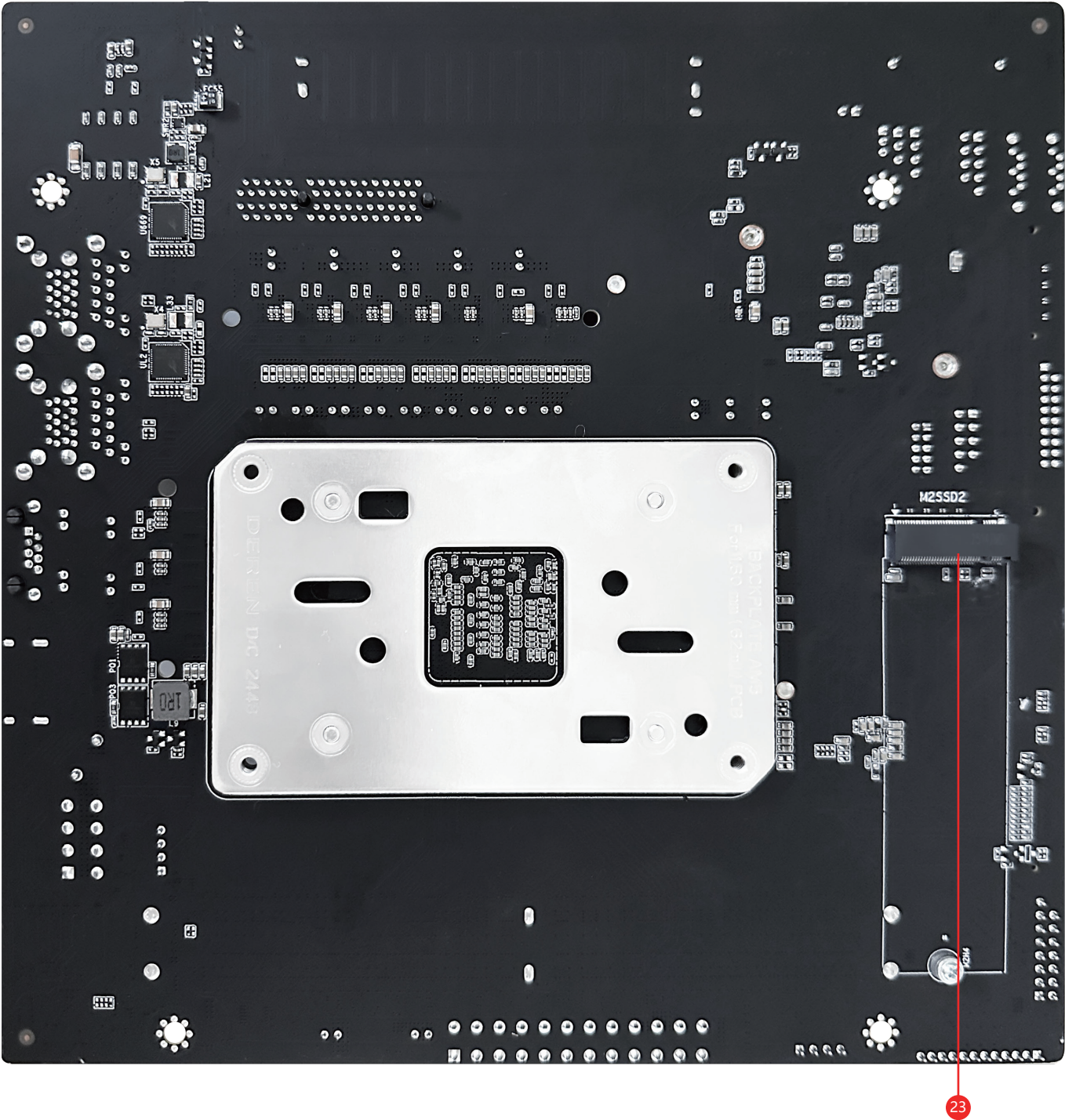
23 M.2 SSD2 slot
